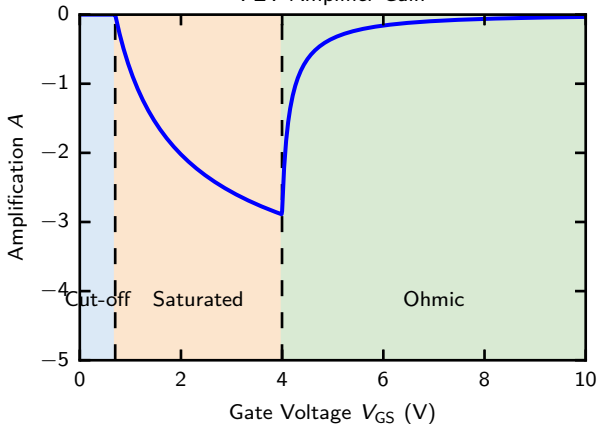
FET Amplifier Gain
